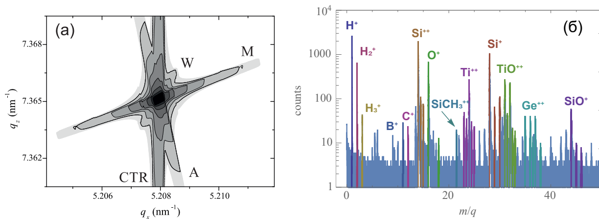
(a) Моделирование сигнала в рентгеновской дифрактометрии высокого разрешения с учетом инструментальных эффектов. Представлена карта обратного пространства для брэгговского отражения 224 кристалла кремния с нормалью, ориентированной в направлении (001). Конфигурация дифрактометра включает монохроматор Ge(004)x4 и анализатор Ge(220)x2. CTR — полоса, обусловленная влиянием границы образца; M — полоса монохроматора; A — полоса анализатора; W — полоса длины волны. (б) Идентификация пиков в масс-спектре атомной зондирующей томографии для полупроводникового устройства из кремния с использованием байесовского подхода. Подписи указывают идентифицированные паттерны ионов.
