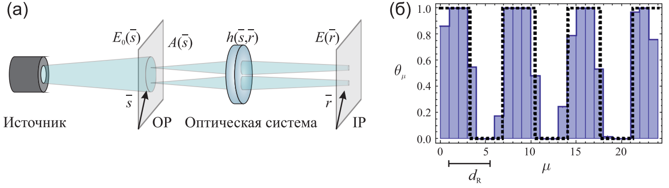
(а) Общая схема измерения в квантовой микроскопии. Увеличенное изображение объекта с амплитудой пропускания A(\vec{s}) , помещенного в объектную плоскость ОР и освещенного источником излучения с известными свойствами, формируется оптической системой с функцией Грина h(\vec{s}, \vec{r}) в плоскости изображения IP. (б) Пример реконструкции амплитуды пропускания модельного объекта (трех непрозрачных полос на прозрачной мишени, освещенной бифотонами) на основе измеренного корреляционного изображения второго порядка. Отрезок в нижней части гистограммы указывает рэлеевский предел разрешения, пунктирные линии — ожидаемую форму модельного объекта.
